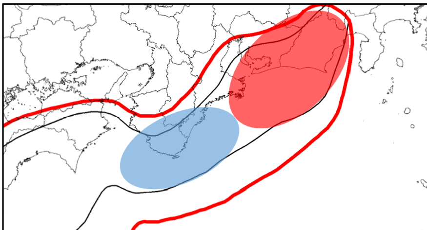
破壊域が昭和東南海地震より西側にある場合
