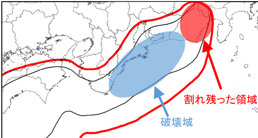
昭和東南海地震
