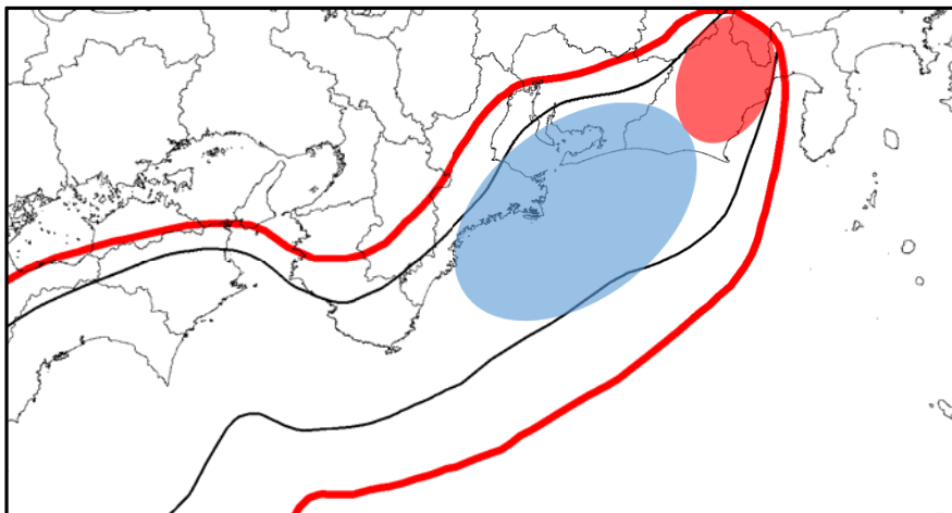
破壊域が昭和東南海地震より東側にある場合
