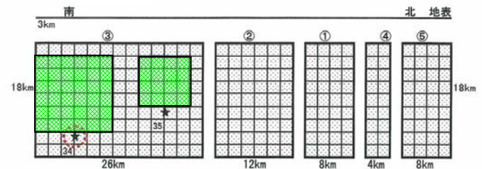
上町断層帯ケース4の断層破壊シナリオ
