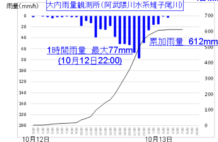
高水時
