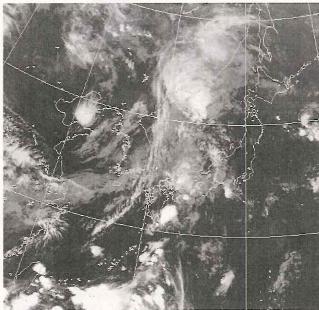
気象衛星画像(赤外) 9月5日09時00分
