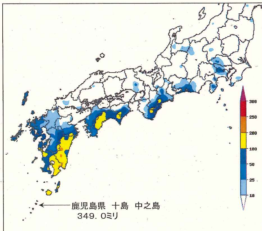
9月1日0時から5日7時までの期間降水量
