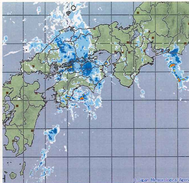
雨雲の状況 9月5日09時00分
