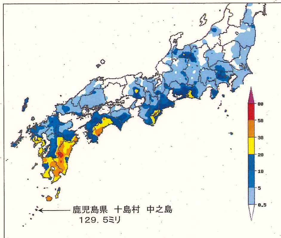
9月1日0時から5日7時までの最大1時間雨量
