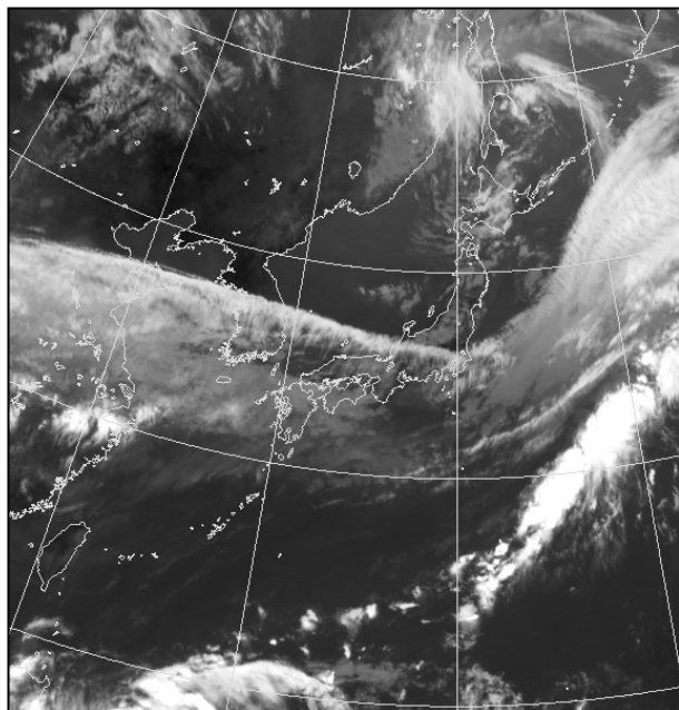
衛星画像(赤外) 9月18日12時
