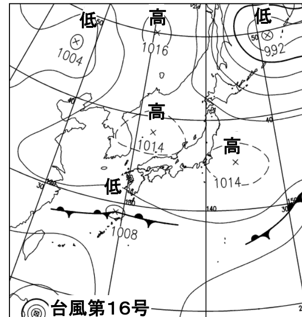
予想天気図 9月19日21時
