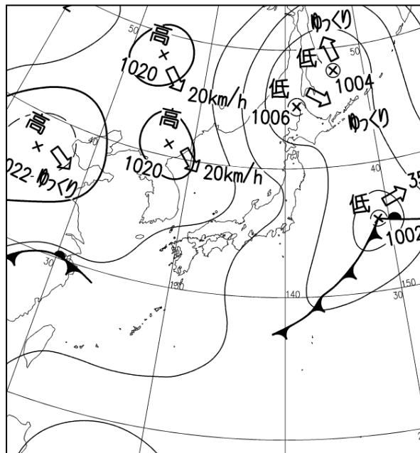
地上天気図 9月18日12時
