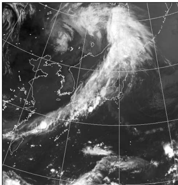
衛星画像(赤外) 9月4日12時
