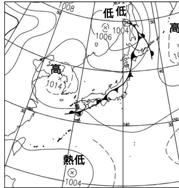
予想天気図 9月5日21時
