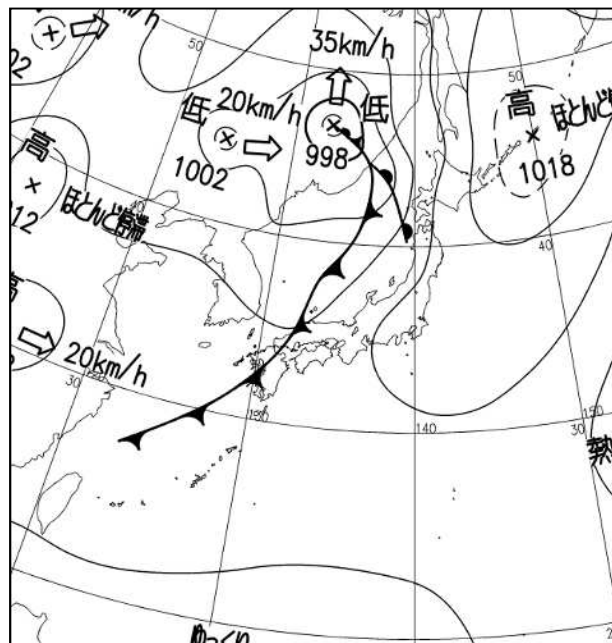
地上天気図 9月4日12時
