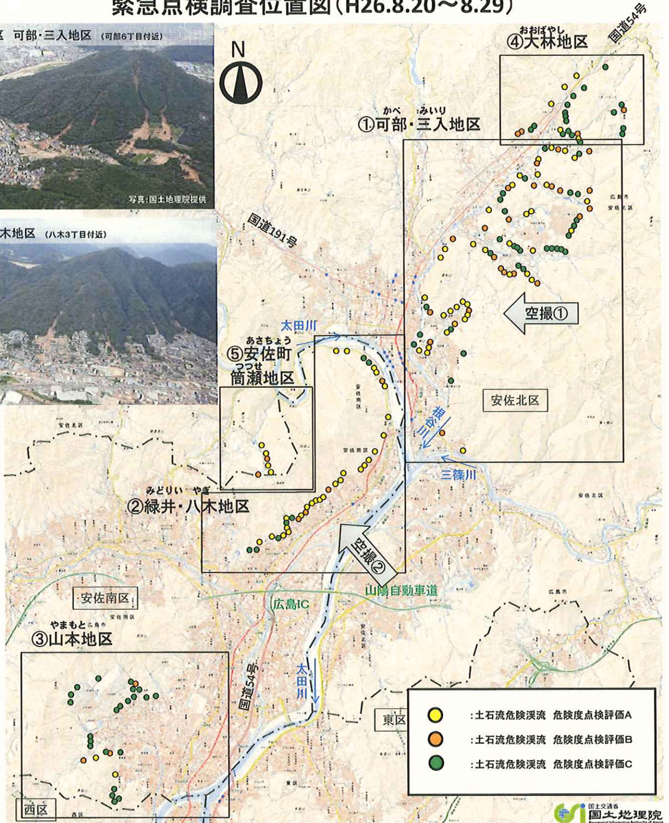
TEC-FORCEによる渓流点検箇所
